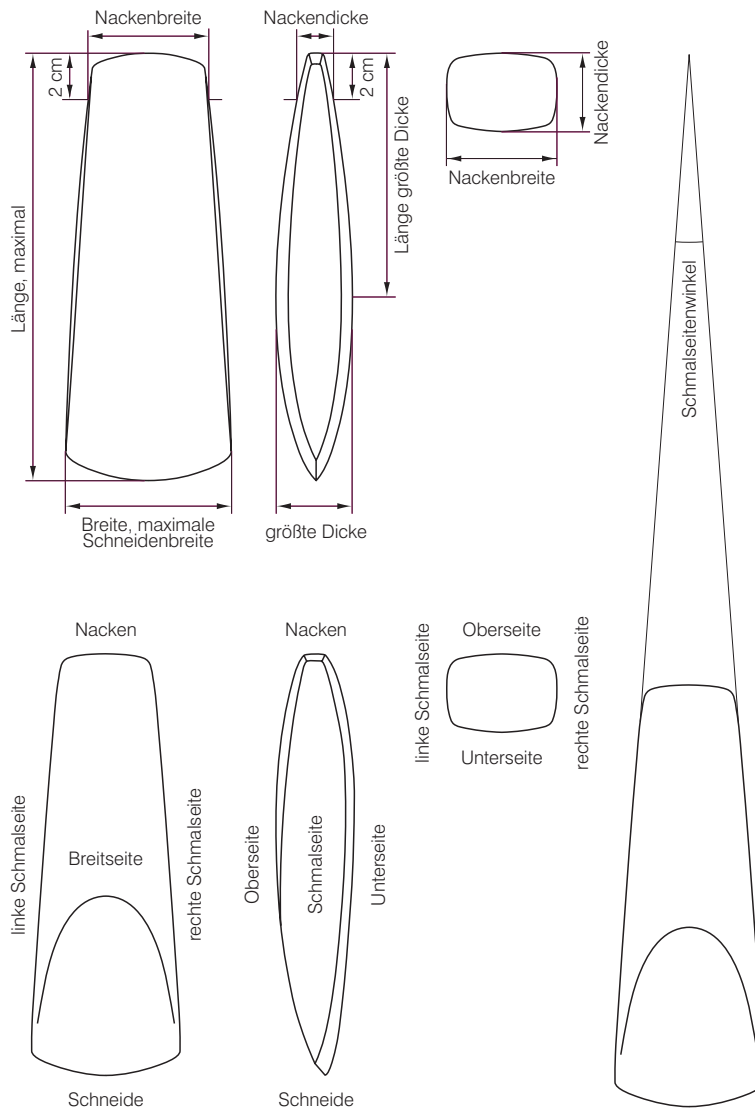
Abb. 4: SDS. Bezeichnung der einzelnen Bauteile (nach Malmer 1962, 360 und Nielsen 1977, 63).
